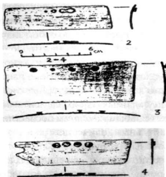
Рис. 4. Пластинки крытого доспеха из Луцка (по С. Терському).
